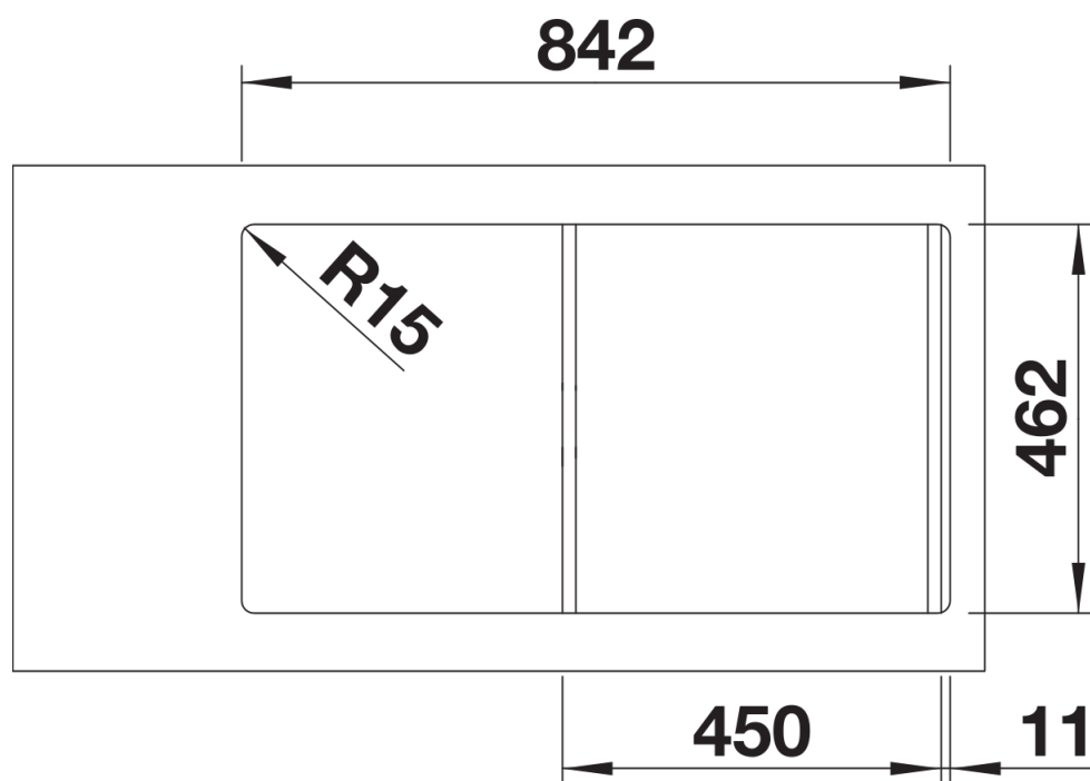
Kivágás
