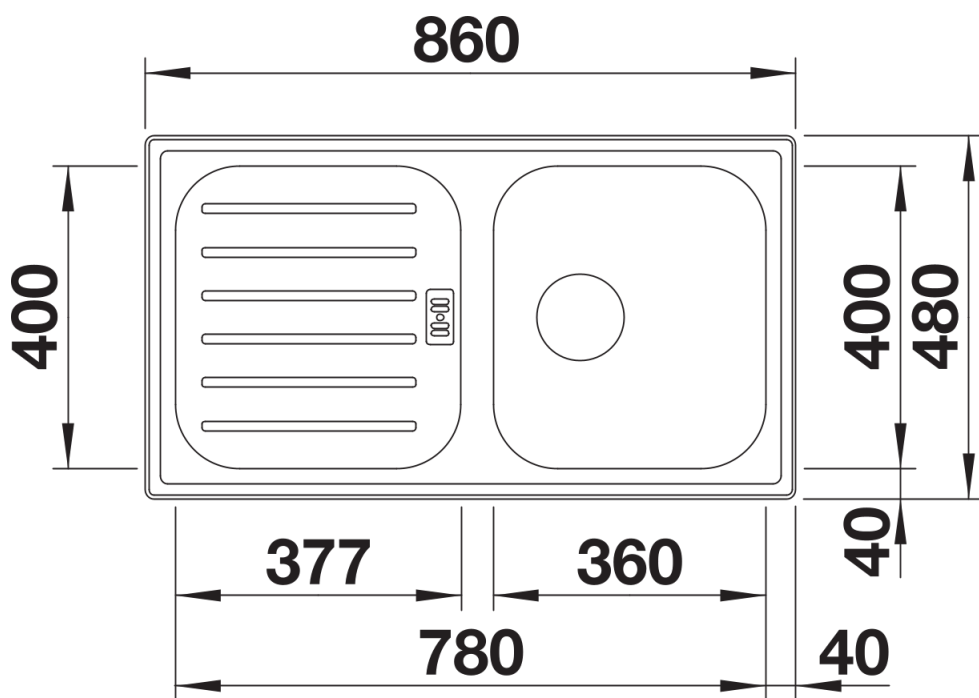
Felülnézet
